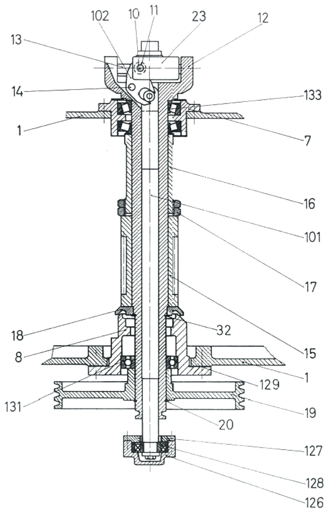
主軸部 分解図
